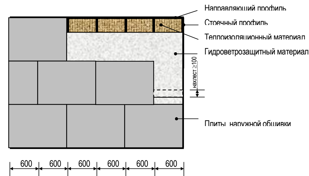
Рис. 16. Крепление наружной обшивки к каркасу
