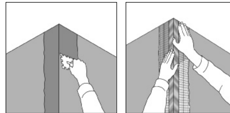
Рис. 21. Армирование углов
