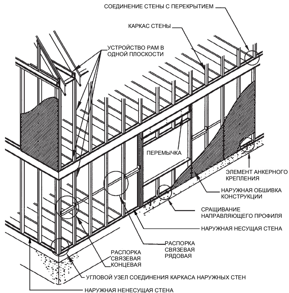
Рис. 2. Стальной каркас стен
