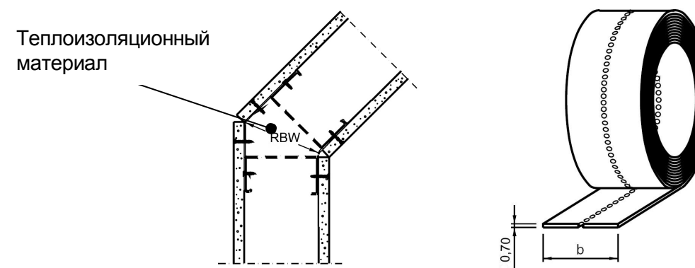
Рис 10. Соединение стеновых панелей под произвольным углом
