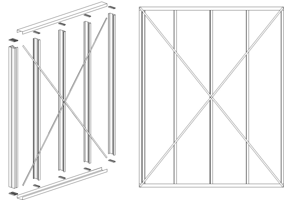
Рис. 5. Каркас панели стены
