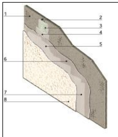
Рис. 18. Декоративное оштукатуривание наружной обшивки
