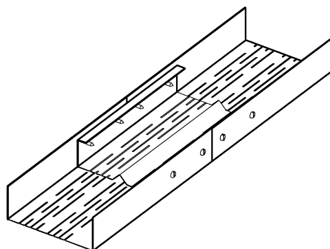
Рис 6. Соединение элементов при помощи «вставок»
