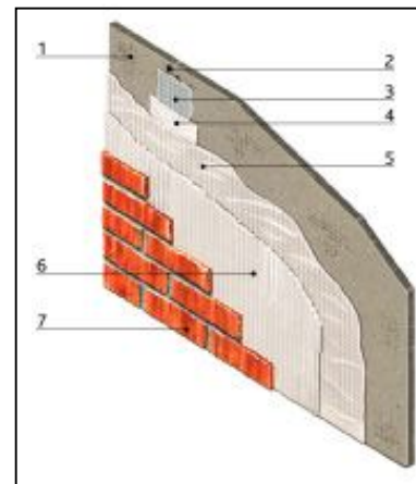
Рис. 20. Облицовка плиточным материалом наружной обшивки
