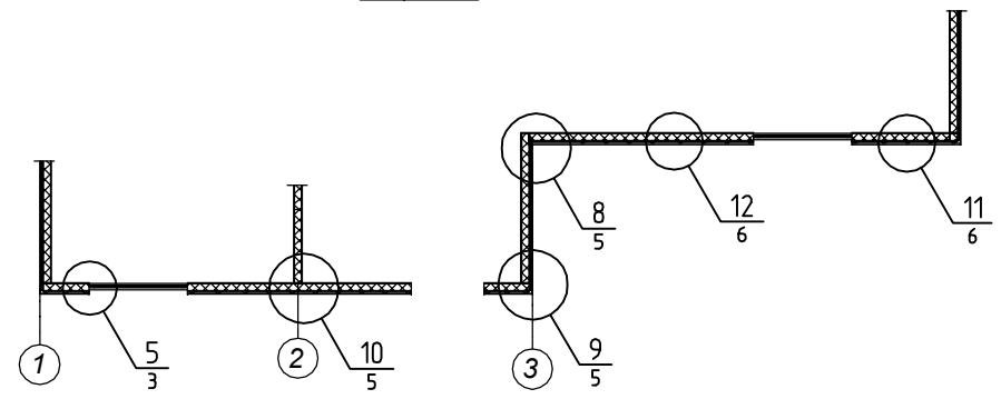
Разрез 1-1
