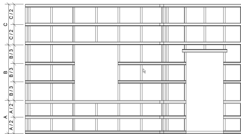
Рис 9. Монтажная схема горизонтальной обрешетки для стен типа 1
