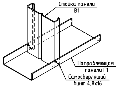
Узел крепления стойки к направляющей.
