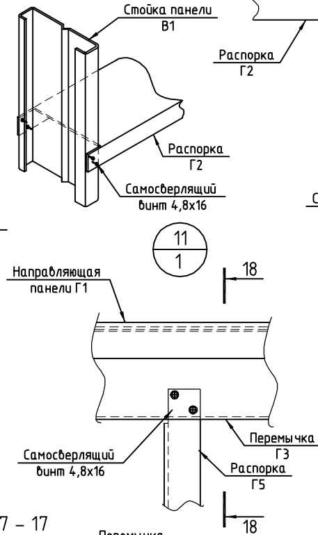
Узел крепления распорки к стойке
