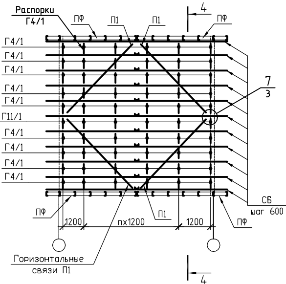
Схема расположения стропильных ферм и распорок и связей
