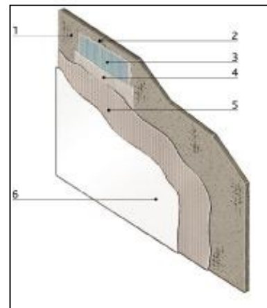
Рис. 19. Окрашивание наружной обшивки
