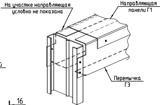
Узел крепления перемычки
